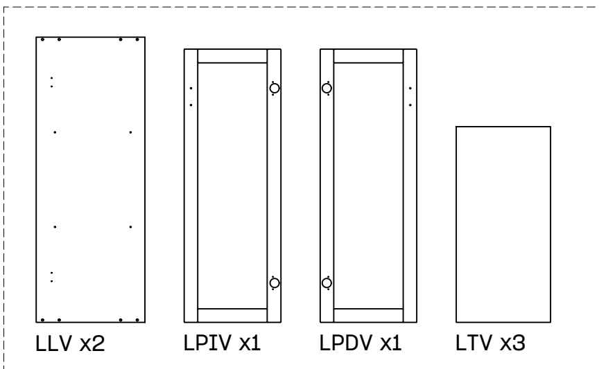
Libe estructura vitrina 2/1 x1
